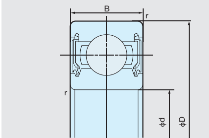
Berührende Dichtscheibe (NSE9)
