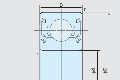
Berührungsarme Dichtscheibe (NKE9)
