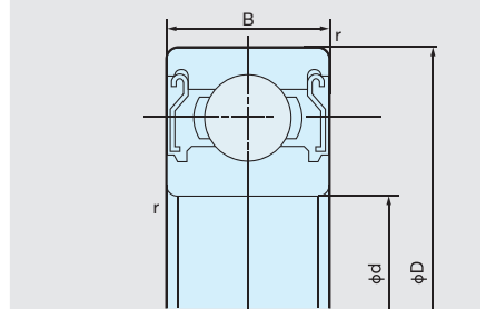
Deckscheibe (ZE)
